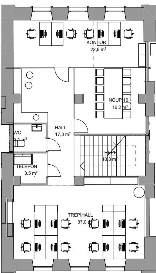
2. korrus
