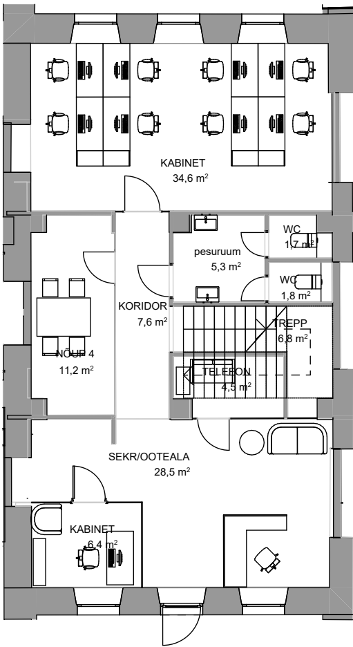
1. korrus
